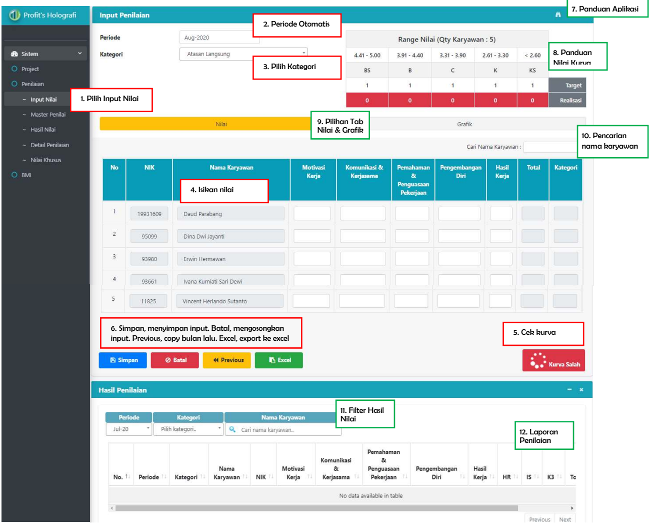
Gambar 3. Halaman Input
